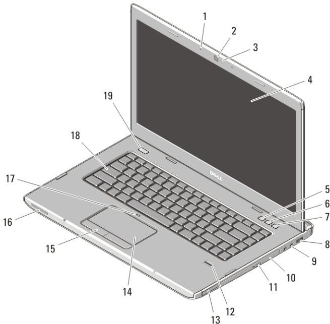
Abbildung 5. Vostro 3550 — Vorderansicht
