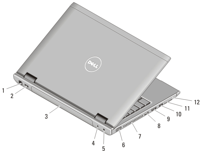
Abbildung 4. Vostro 3450 — Rückansicht
