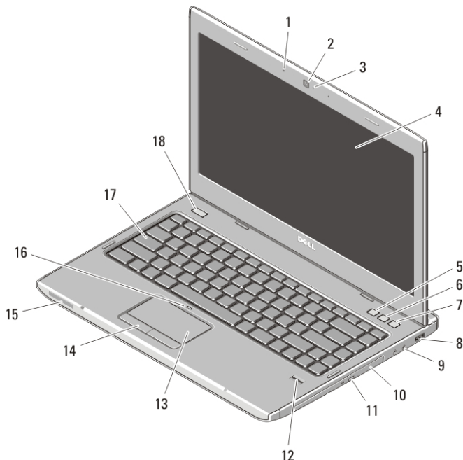
Abbildung 3. Vostro 3450 — Vorderansicht
