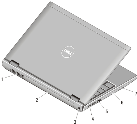
Abbildung 2. Vostro 3350 — Rückansicht
